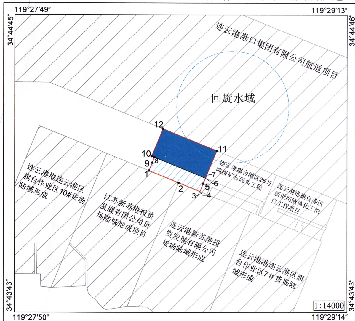
连云港港旗台作业区矿石码头改扩建工程宗海界址图
